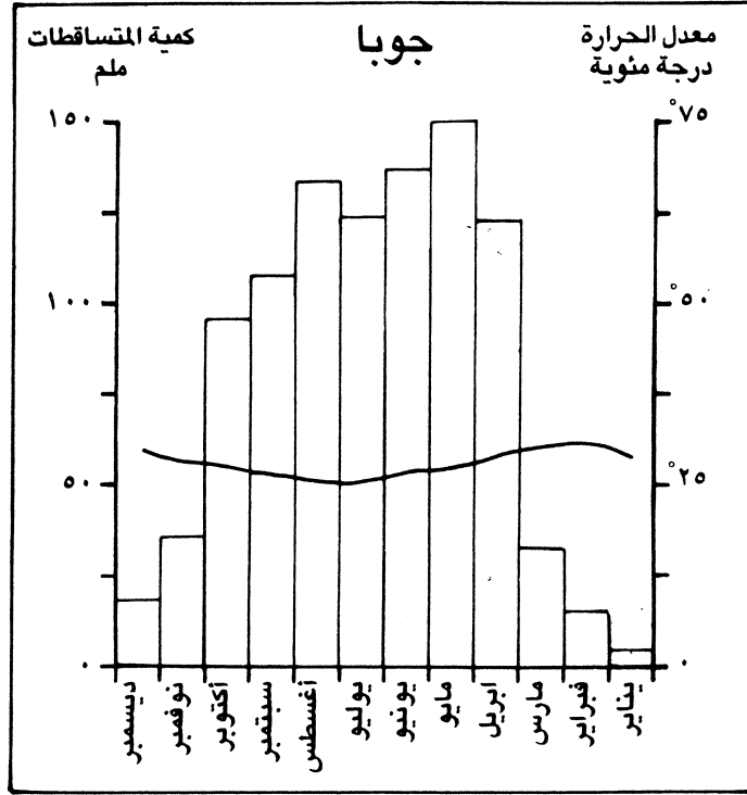
رسم بياني مناخي لمحطة جوبا المناخية في جنوب السودان
