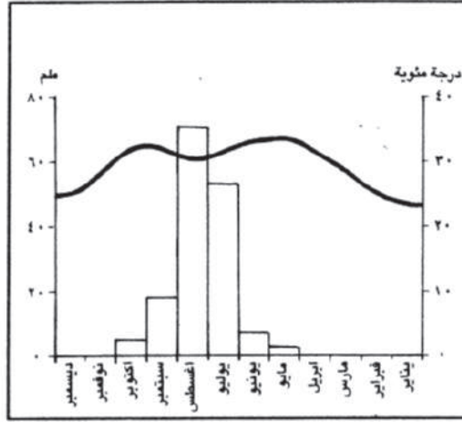
رسم بياني لمحطة الخرطوم المناخية
