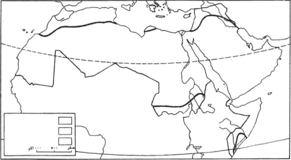
خريطة الوطن العربي المناخية
