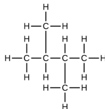
3,2 - ثنائي ميثيل بيوتان
