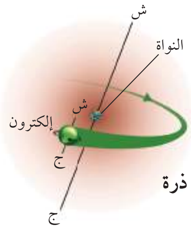
الشكل ٤ تولّد حركة الإلكترونات في الذرة مجالات مغناطيسية.
