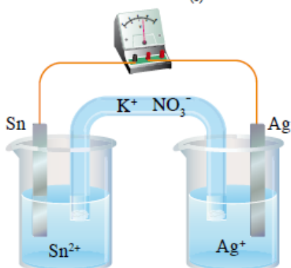
الشكل (٢-٤): خلية غلفانية قطبها Sn و Ag.
