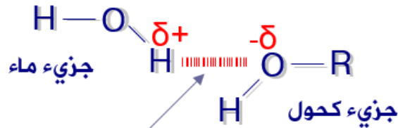
رابطة هيدروجينية
