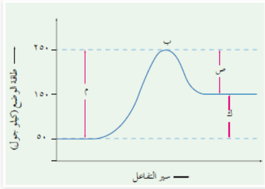
الشكل (٣-١٥): منحني طاقة الوضع أثناء سير التفاعل.
